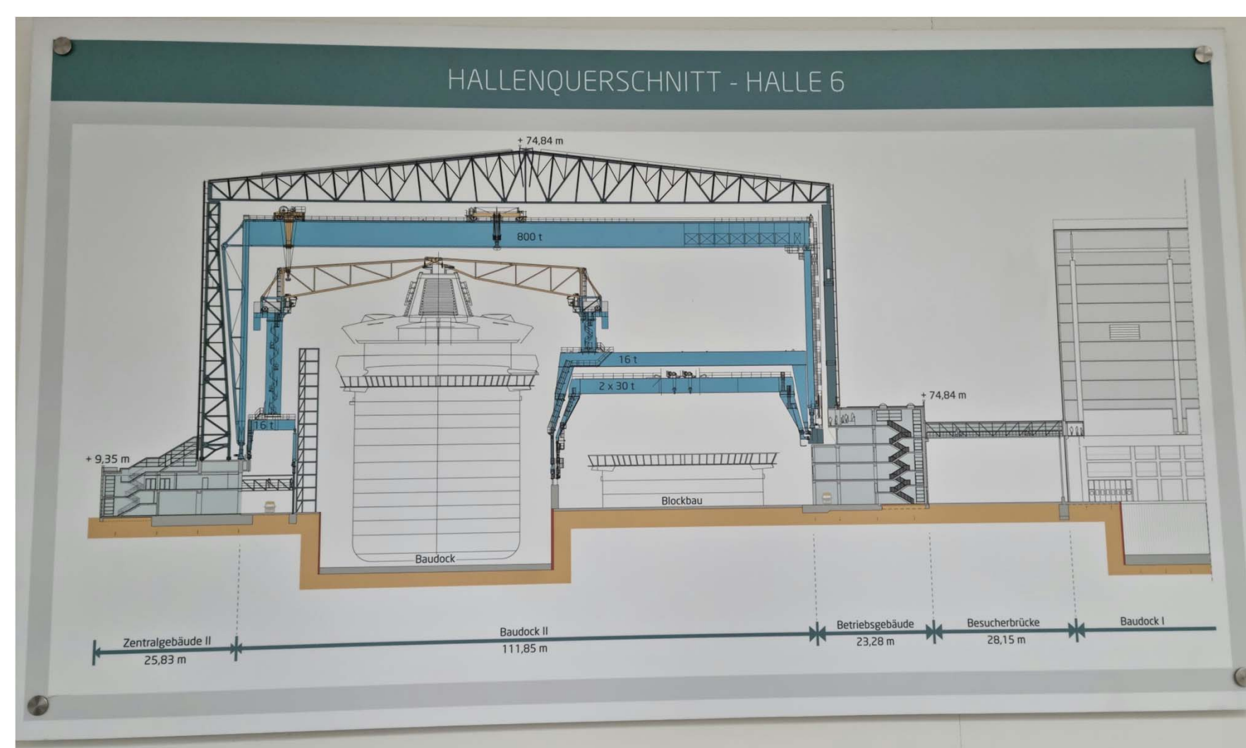
Hallenquerschnitt von einer Werfthalle
